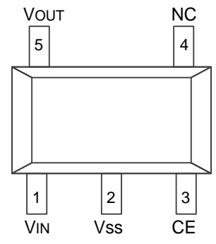
SOT23-5
